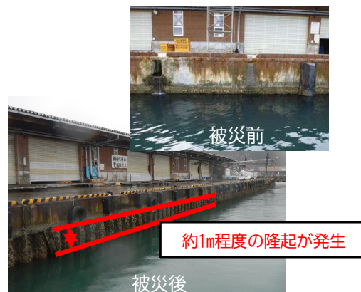
船だまりの被害状況
