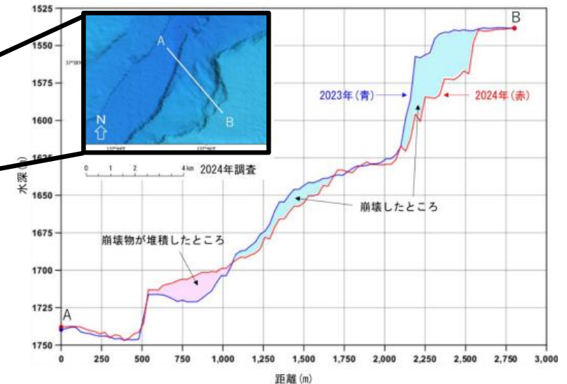
図2 2023年5月と今回(2024年2月)の海底地形の比較【断面図】
