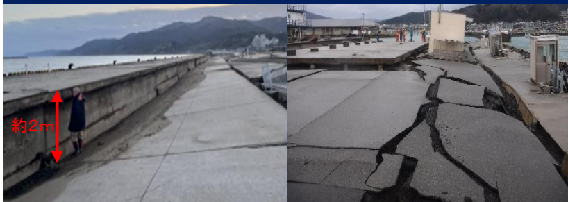
岸壁背後の沈下
