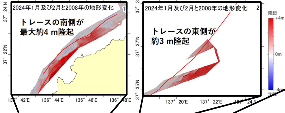
図1 2008年と今回(2024年)の海底地形の変化量(赤線は活断層トレース)
