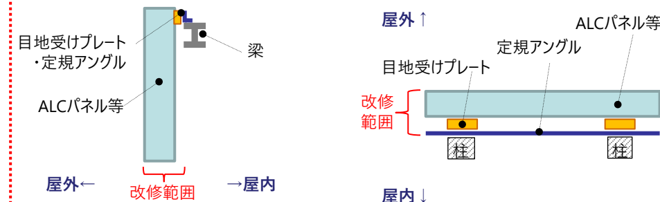
図2-7 横から見た断面図
