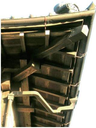
写真 2-8 せがい造り
