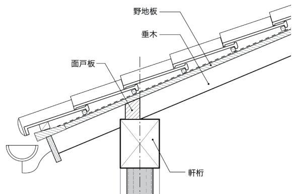
図 2-11 面戸板現し
