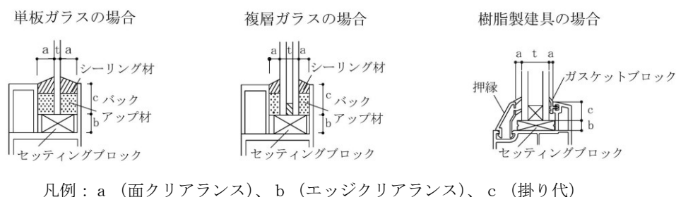
図 16.14.1 ガラス溝
