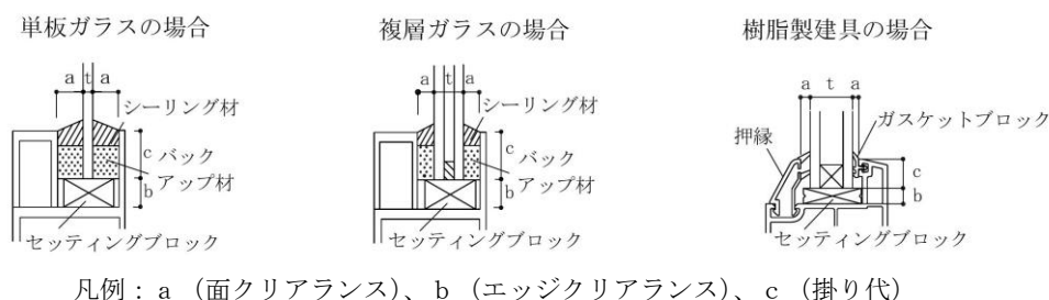
図 5.14.1 ガラス溝
