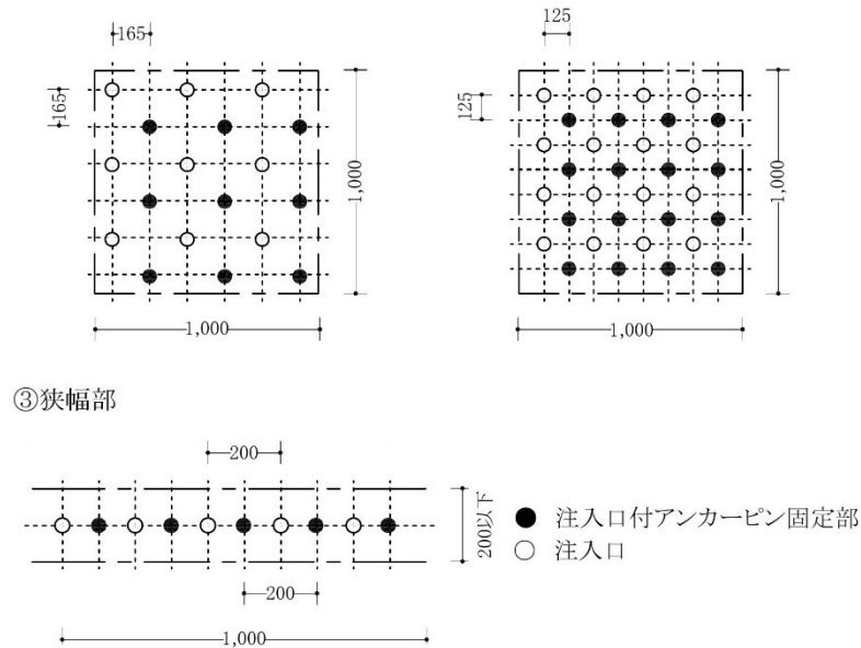
①一般部分標準グリッド(165×165) ②指定部分標準グリッド(125×125)
