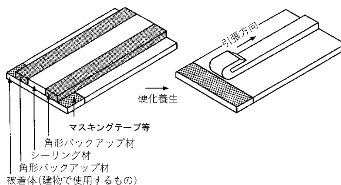
図 3.7.1 簡易接着性試験
