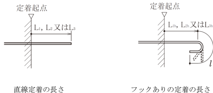
図 8.3.2 直線定着の長さ及びフックありの定着の長さ
