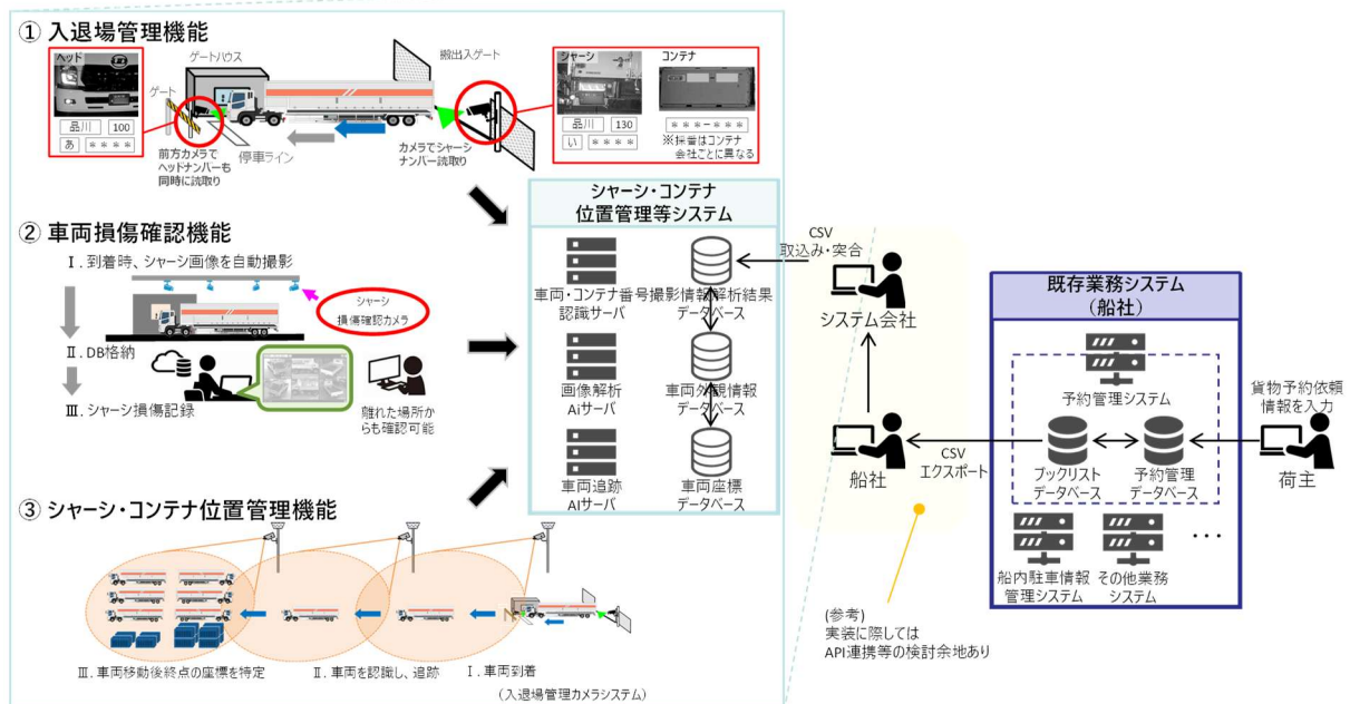
図 4-2 現地技術検証に用いたシャーシ・コンテナ位置管理等システムの概要
