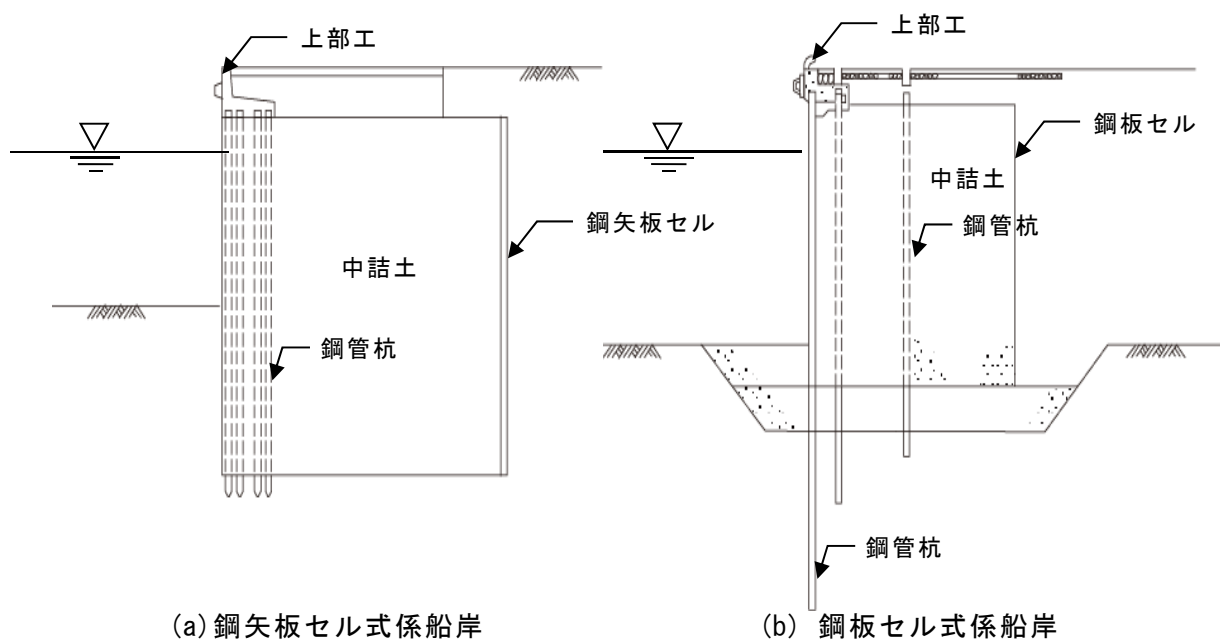
図 3-6.7 鋼矢板セル式係留施設の断面図の例
