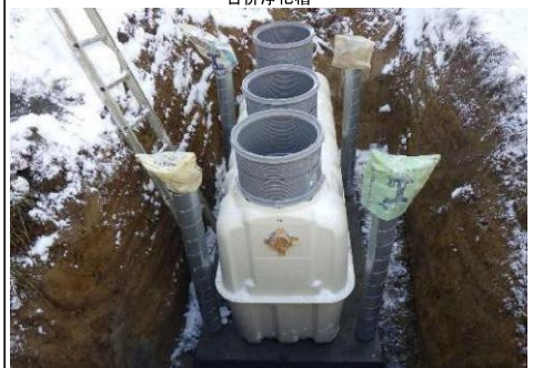
施工状況
