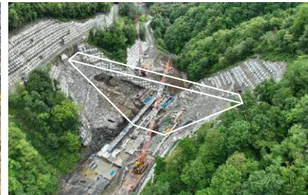
幾春別川総合開発事業 (三笠ぼんべつダム(三笠市))
