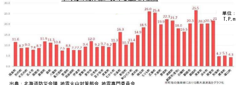
市町毎の海岸線における最大津波高
