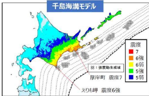
千島海溝や日本海溝周辺で発生が想定される最大クラスの地震の震度分布
