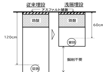
凍結深さを考慮した浅層埋設のイメージ
